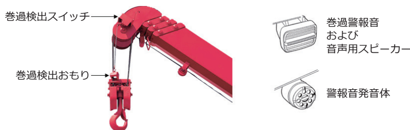
図1-48 巻過警報装置
