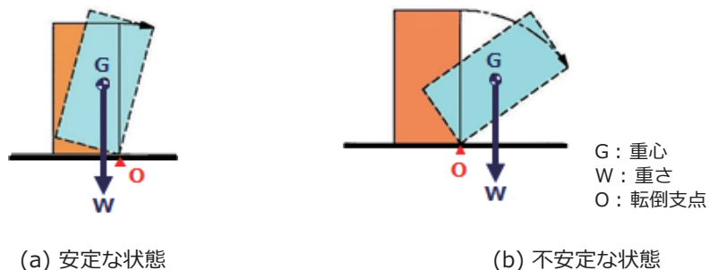
図3-9 物体の安定
