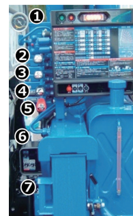
図1-19 積載形トラッククレーンの 操作レバー・スイッチ例
