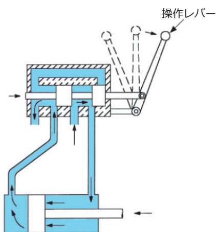
図2-11 方向切換弁
