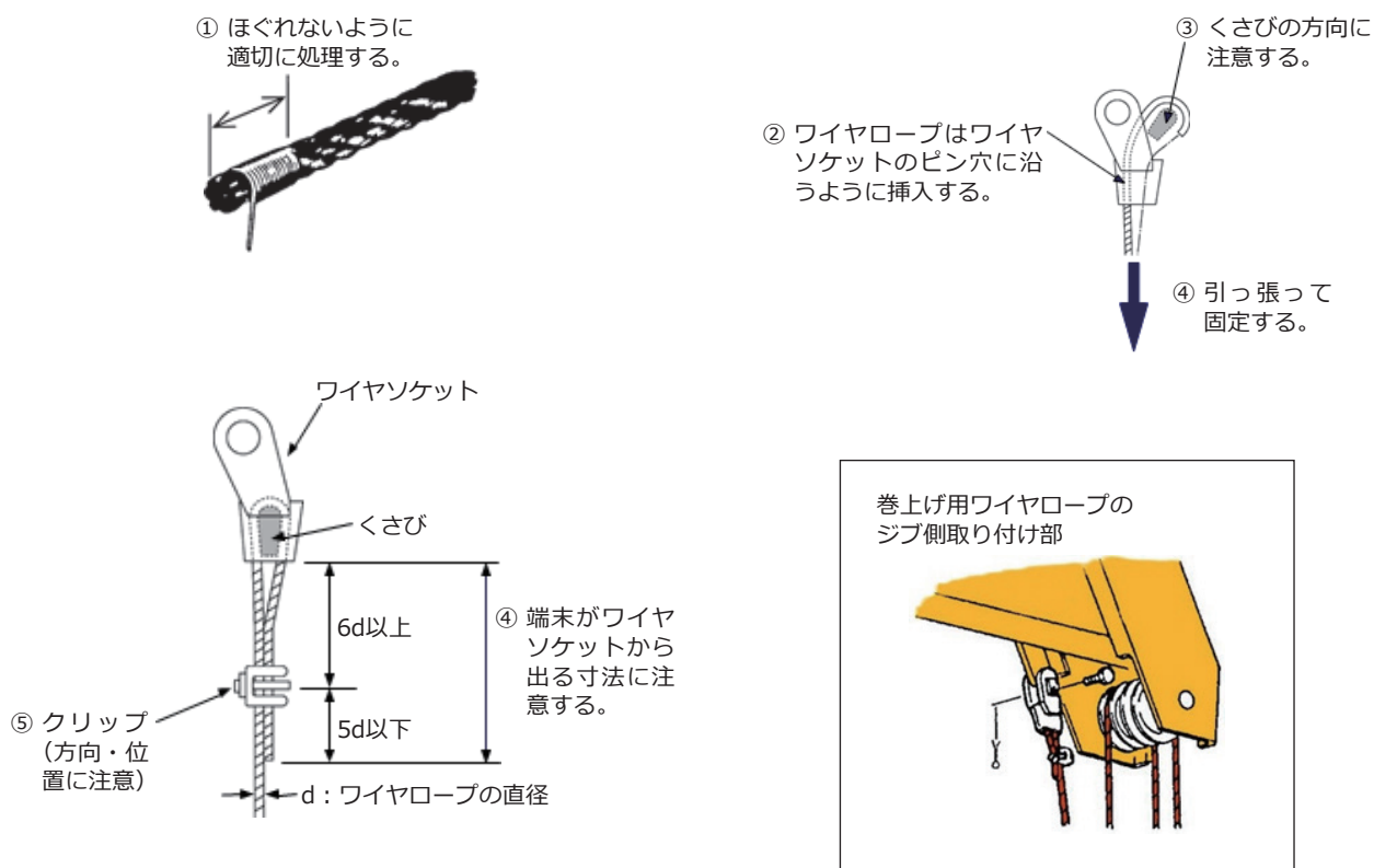
図1-89 ジブ側の端末処理
