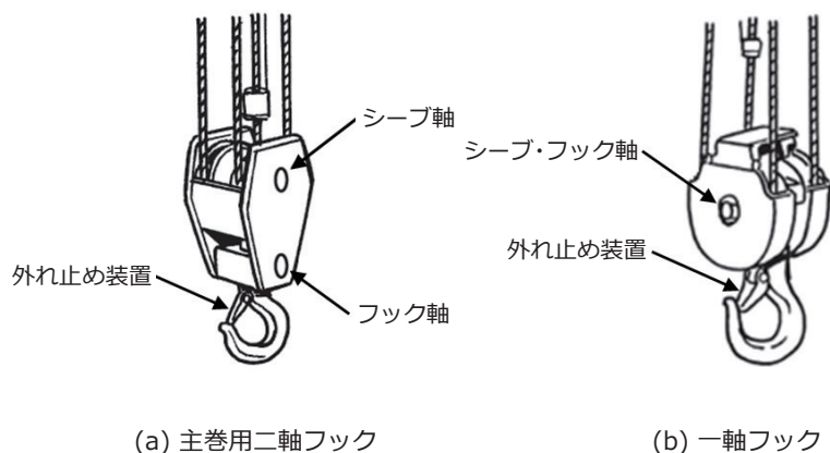
図1-43 主巻フック
