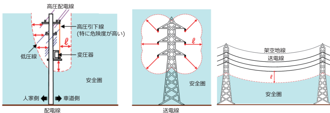
図2-17 安全距離(離隔距離)(図中の l は危険範囲)
