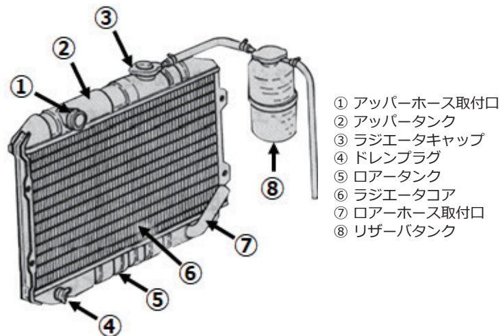
図2-2 ラジエータ
