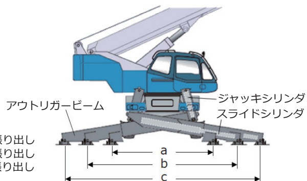
図1-25 X型アウトリガー (ラフテレーンクレーン)
