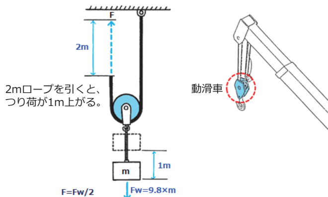
図3-15 動滑車
