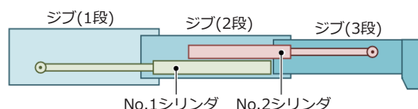
図1-41 3段順次伸縮ジブの構造
