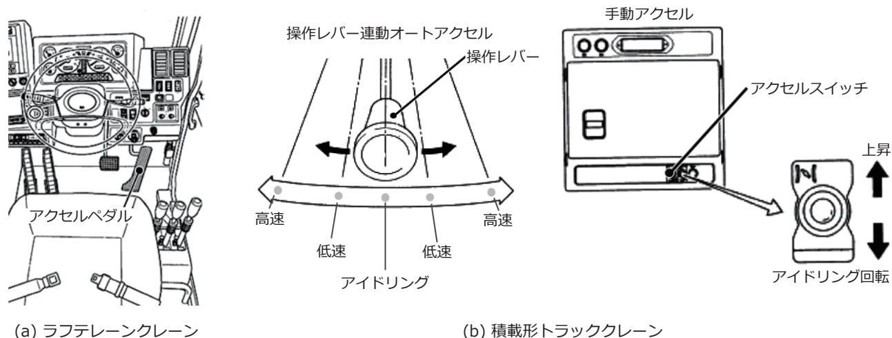
図1-63 アクセル操作
