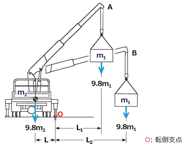
図3-7 積載形トラッククレーンのモーメント
