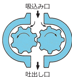
図2-6 ギヤポンプ
