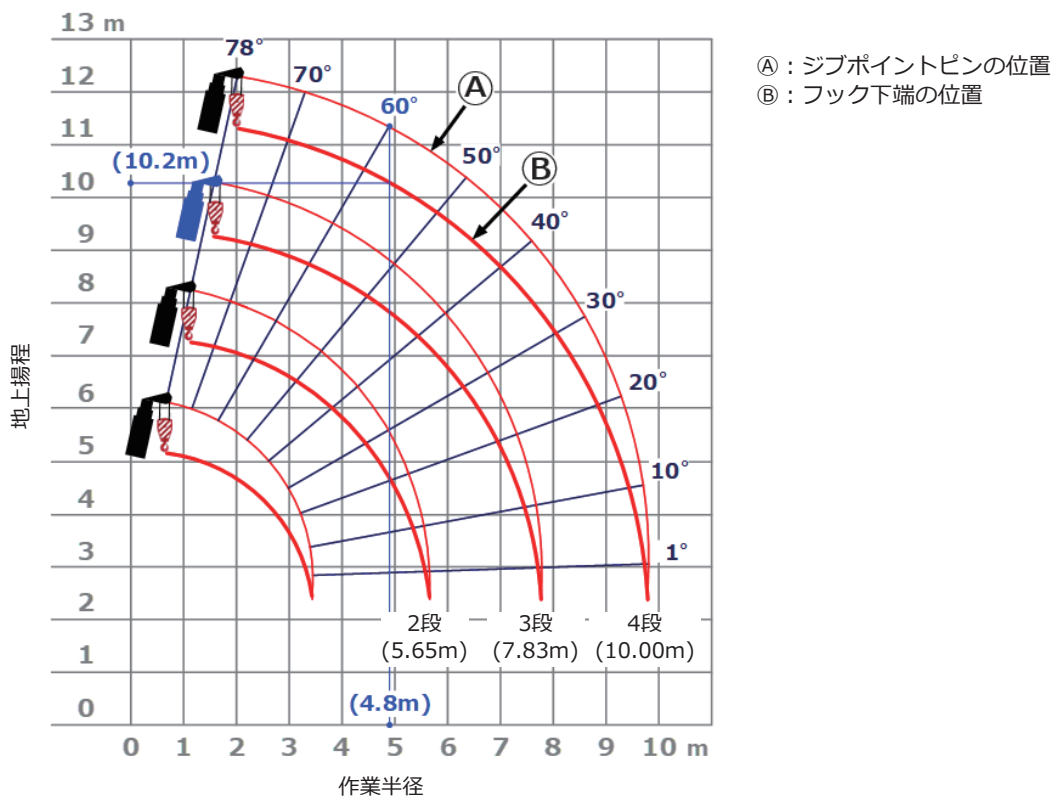
図1-67 積載形トラッククレーンの作業半径-揚程図
