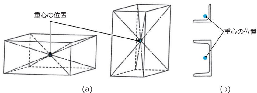
図3-8 重心の位置
