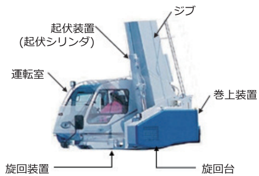
図1-16 ラフテレーンクレーン上部旋回体
