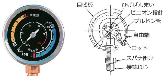
図2-13 圧力計
