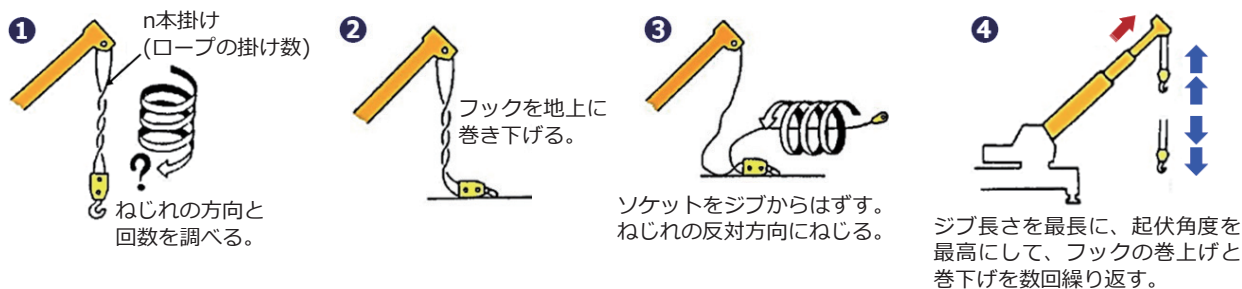
図1-90 巻上げ用ワイヤロープのねじれの取り方
