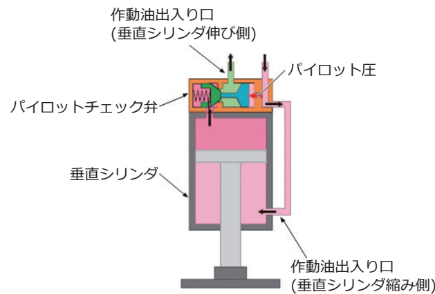
図2-12 パイロットチェック弁
