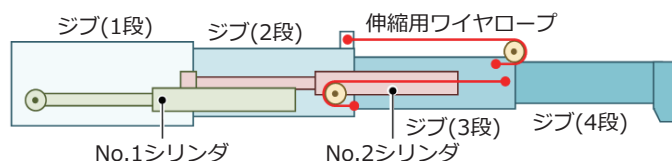
図1-42 4段順次・同時伸縮ジブの構造
