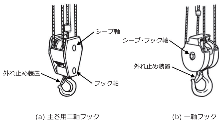
図1-43 主巻フック
