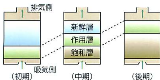
吸収缶の破過と経過
