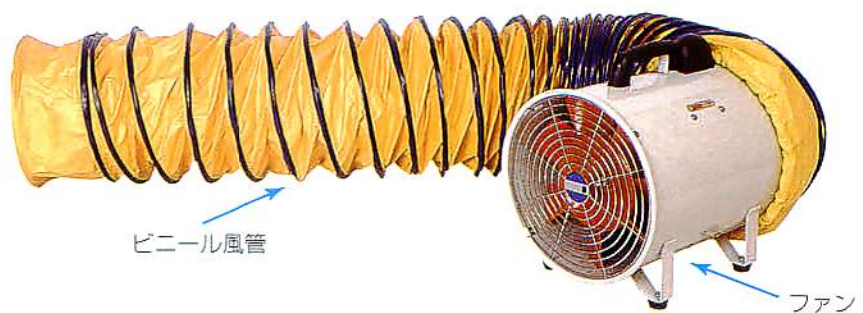
機械換気装置の一例
