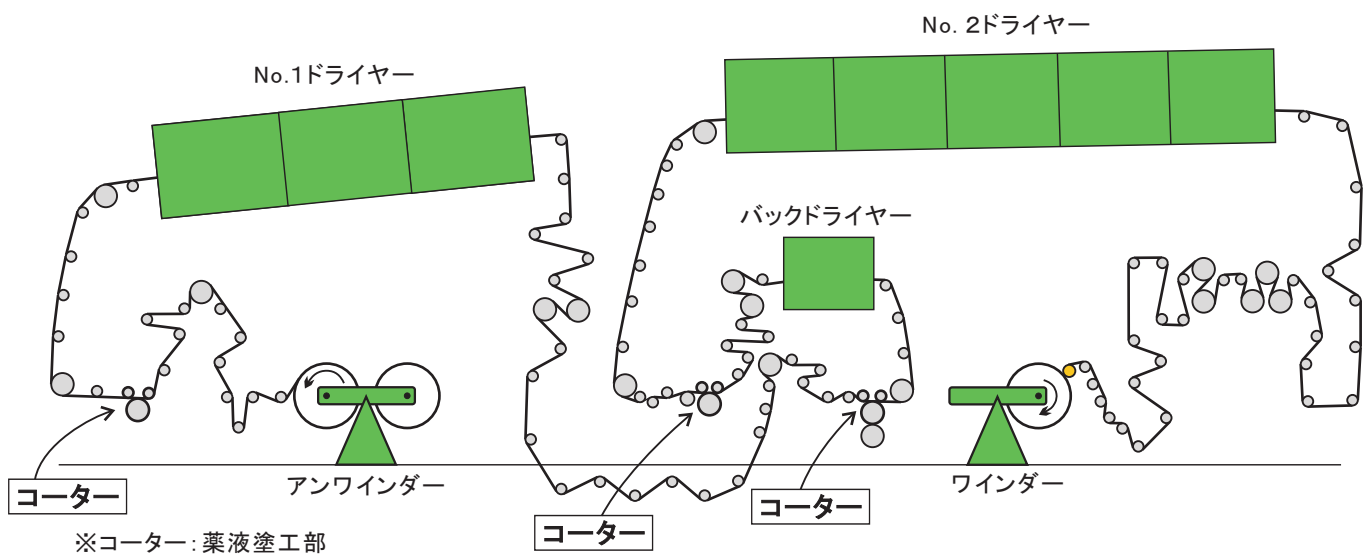
図1 サーマルペーパー塗布工程 全体概要図
