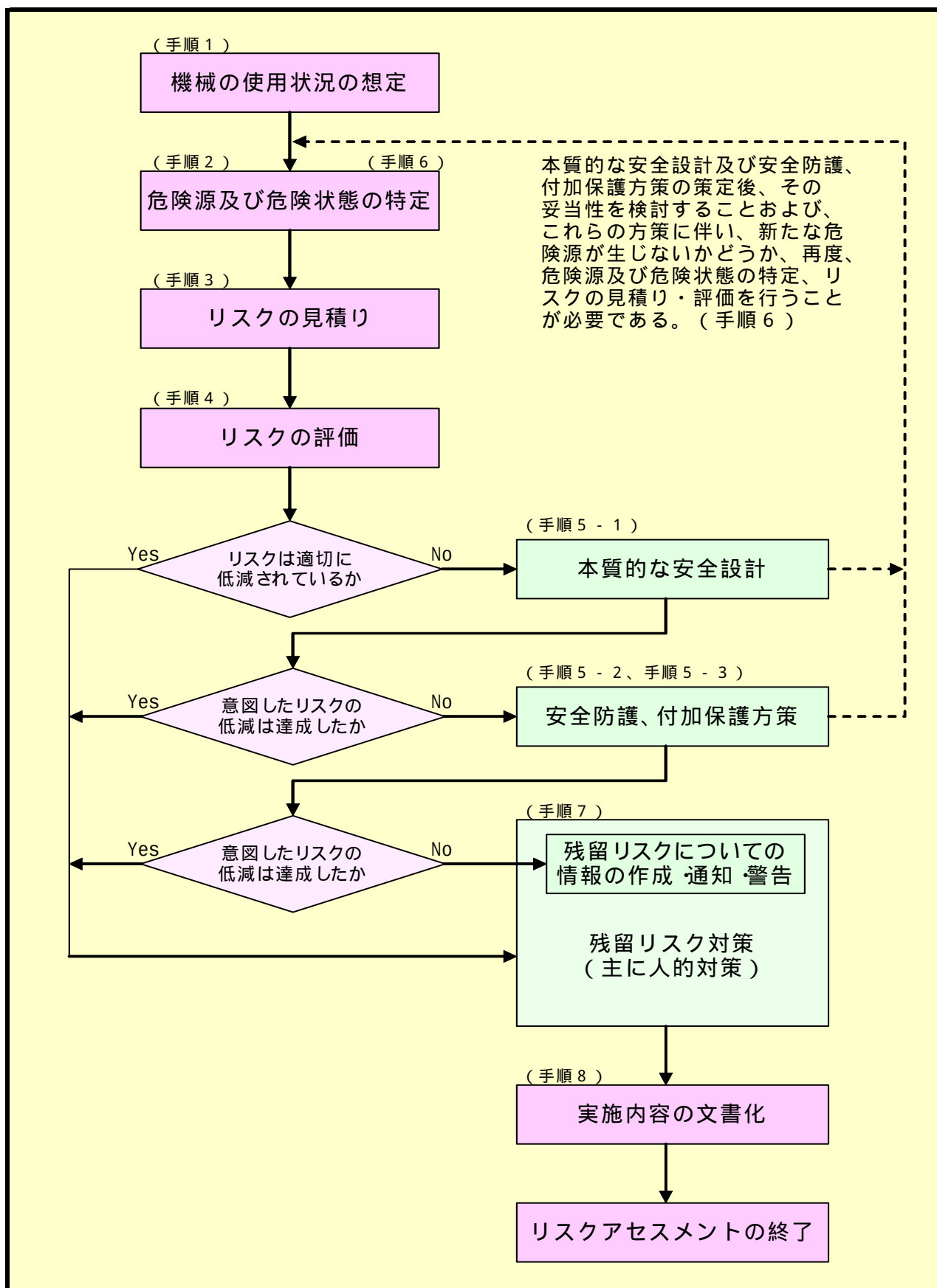
図1 リスクアセスメントと保護方策実施の手順
