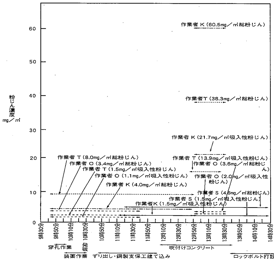
図2-14 B4トンネル工事作業環境測定結果
