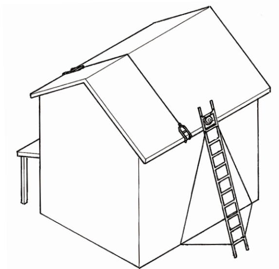
設置の例1（軒先にフック金具を取り付けて主綱を固定する場合）
