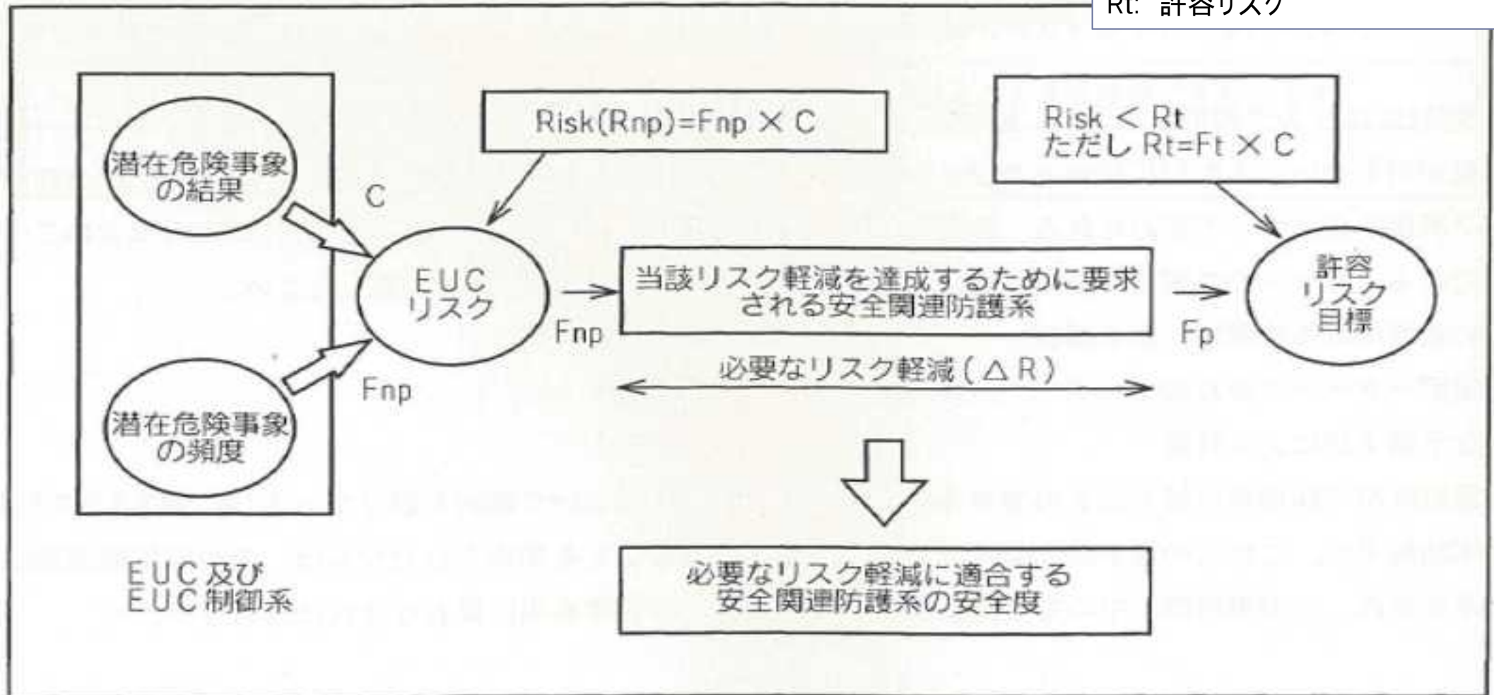
附属書C図1 安全度の割り当て：安全関連防護系の例
