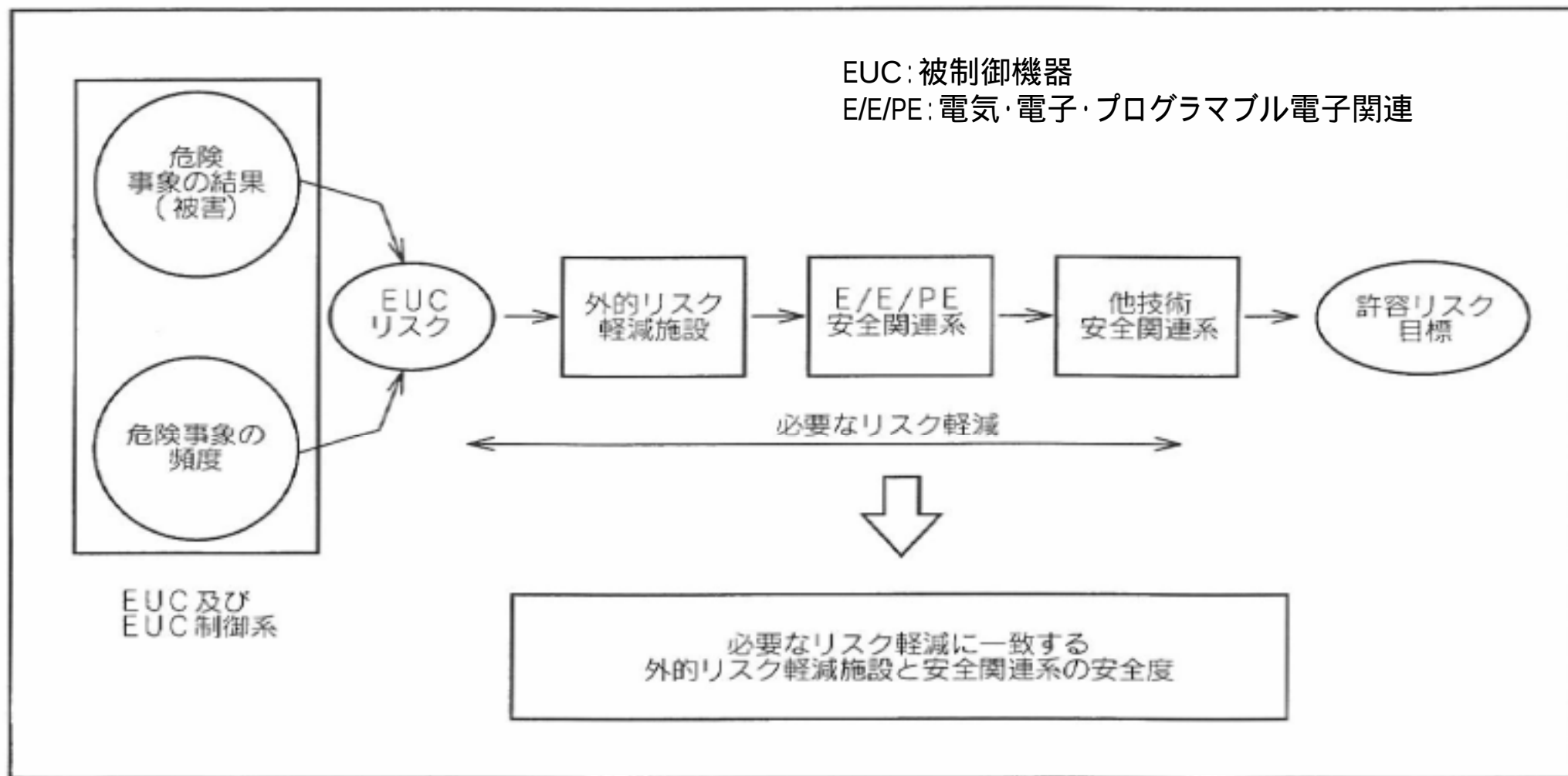
附属書A図2 リスク及び安全度の概念
