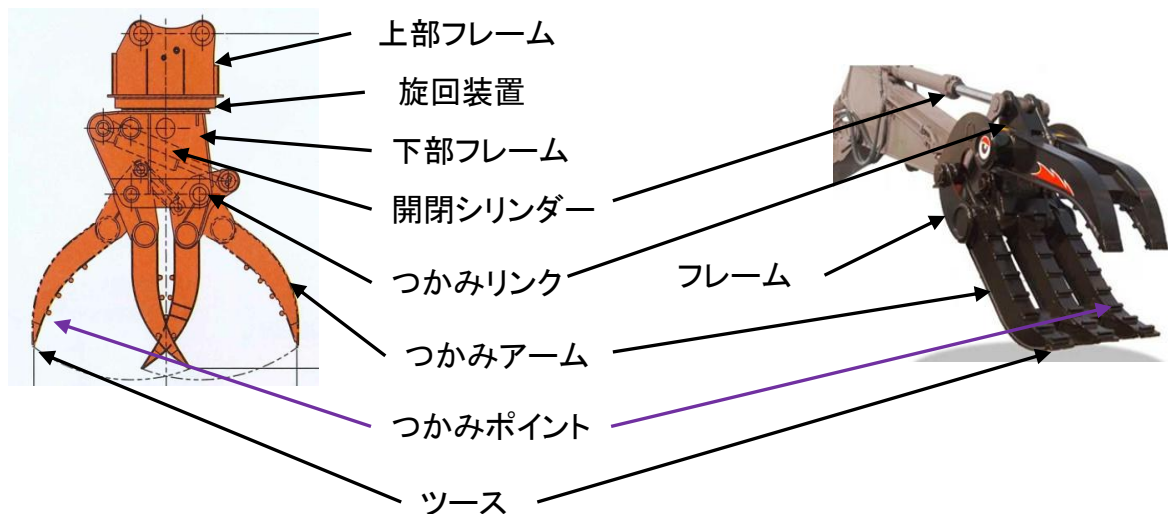
つかみ具(内部シリンダー作動型)
