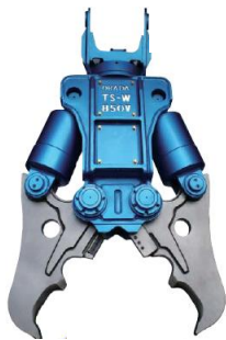
コンクリート圧砕機(大割or小割)
