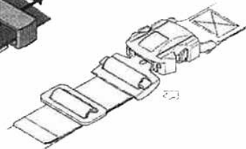
ワンタッチバックルの通し方
