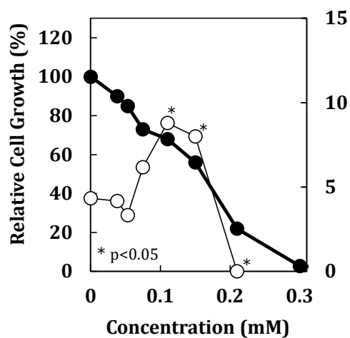
図2 炭酸ジフェニルのBhas 42細胞における形質転換試験(本試験)結果
