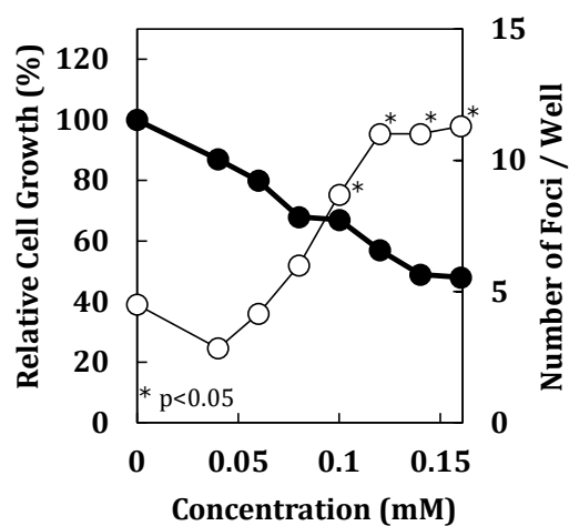
図3 炭酸ジフェニルのBhas 42細胞における形質転換試験(確認試験)結果
