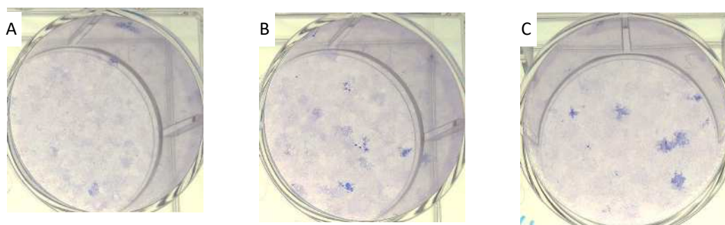
図4 ギムザ染色したBhas 42細胞の代表的ウェル
