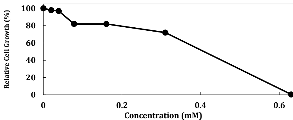
図1 炭酸ジフェニルのBhas 42細胞における細胞増殖試験の結果
