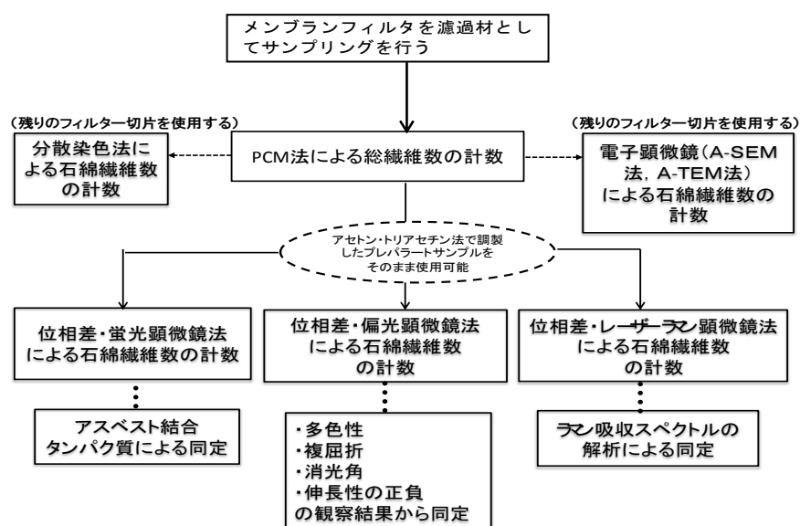
図-26 メンブランフィルタで採取した試料の測定方法
