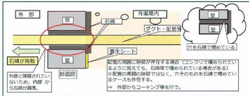
図ー７ 設備ダクト、配管等が壁を貫通している場合の注意事項
