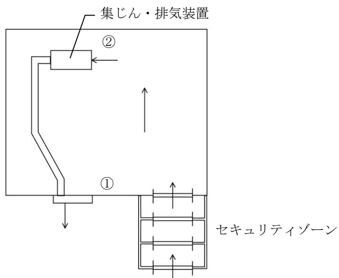
図－８ 集じん・排気装置設置例
