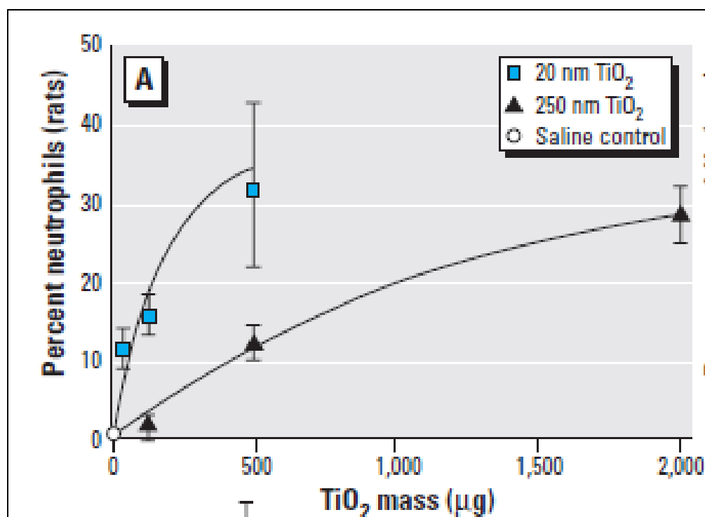
図1 異なる粒子サイズを気管内注入した BALF 好中球比率 –重量基準 (Ferlin et al. 1992、IUCLID 2000)
