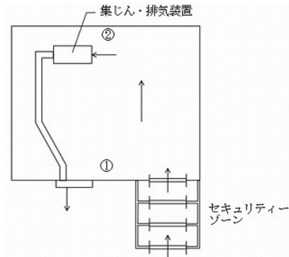
図－8 集じん・排気装置設置例
