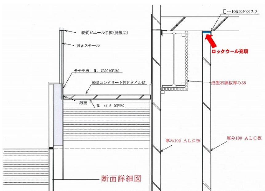
写真Ⅱ－15 スラブ層間塞ぎ図面
