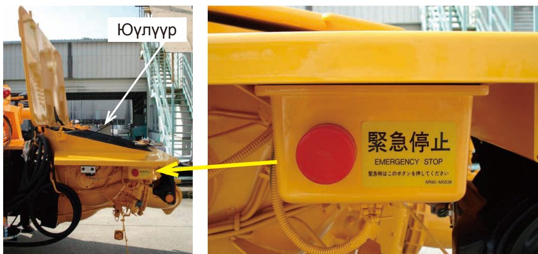
Онцгой үед зогсоох төхөөрөмжийн жишээ
