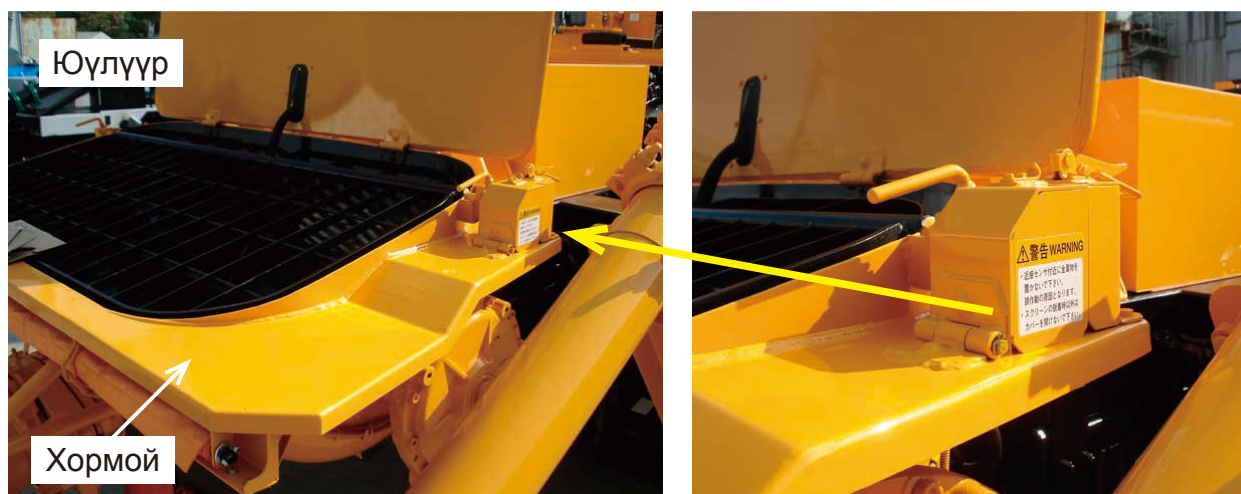
Автомат зогсоох төхөөрөмжийн жишээ
