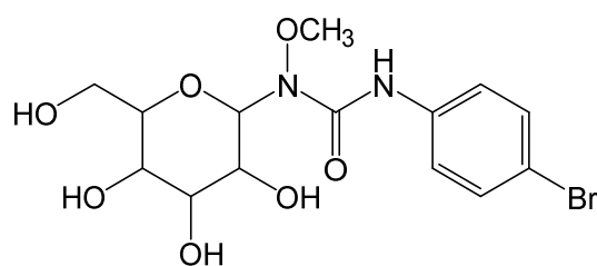
代謝物XVII
