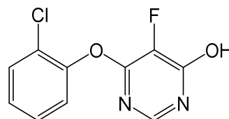
代謝物 M55
