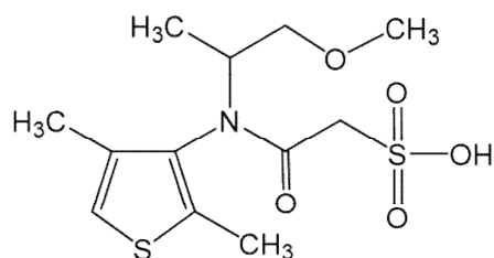
代謝物M27
