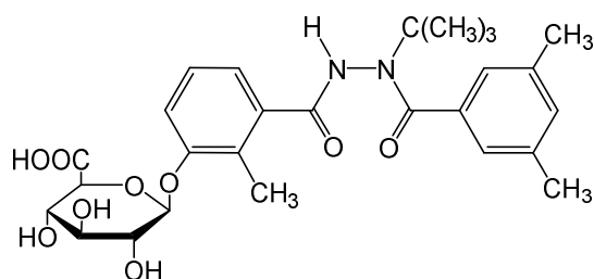
代謝物 L
