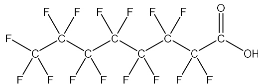
（図1）PFOAの構造例
