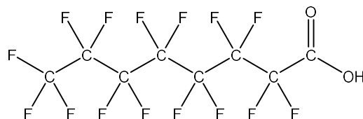
（図１）PFOAの構造例
