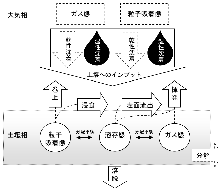
12 図表 V-16 土壌中の化学物質の挙動と物質収支
