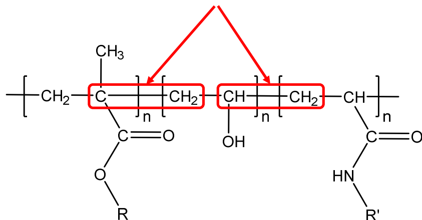
該当する炭素－炭素結合
