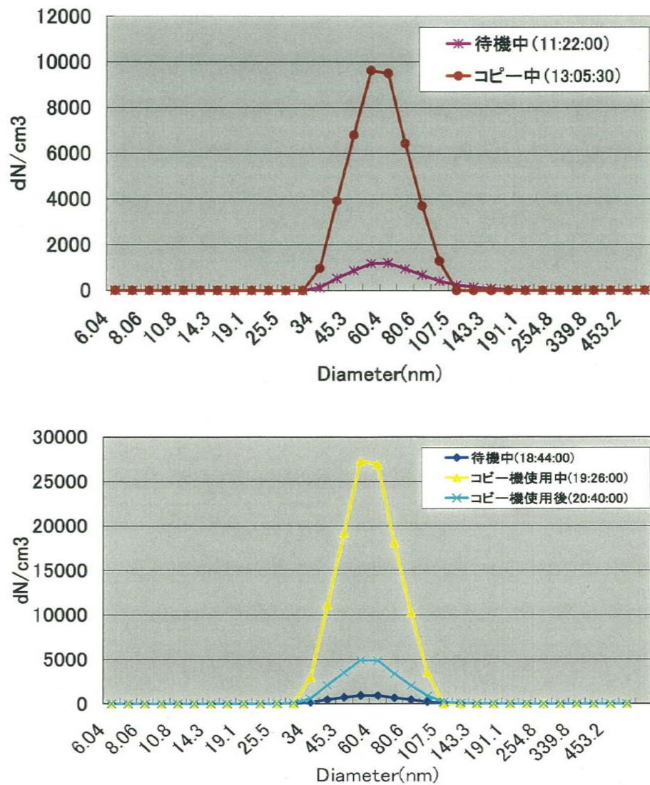
図 1.1.5-6 コピー機からのナノ粒子の拡散に関する測定結果 (測定装置メーカーweb 情報から引用) (上: A4 片面カラーコピー、下: A3 両面カラーコピー)
