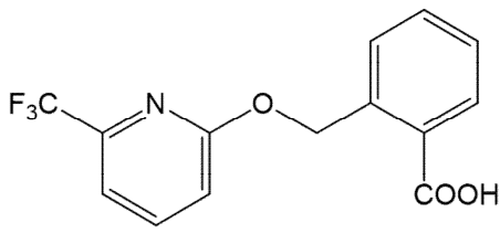
代謝物F
