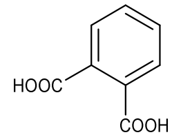
代謝物Z
