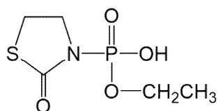
代謝物D
