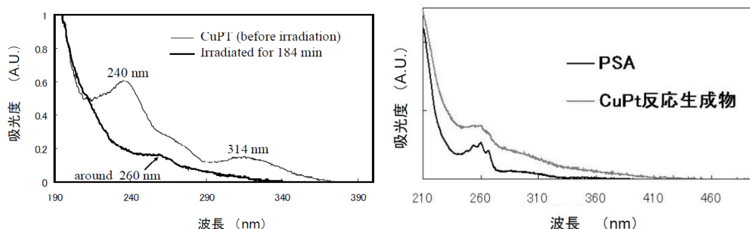
78 図 1-1 千田ら(2005)における銅ピリチオンの光分解産物の同定結果
