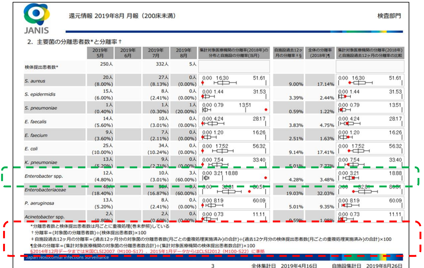
図 7. 検査部門還元情報月報「主要菌の分離患者数と分離率」
