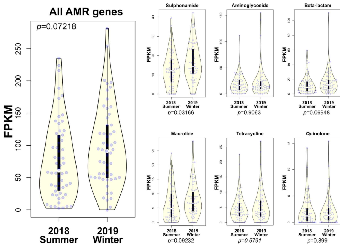
図3 本邦の下水処理場（水再生センター）放流水のメタゲノム解析 (Metagenomic DNA-Seq) 各種カテゴリーの薬剤耐性因子（ARG）の検出量を FPKM（Fragments Per Kilobase of exon per Million mapped fragments）で標準化した。
