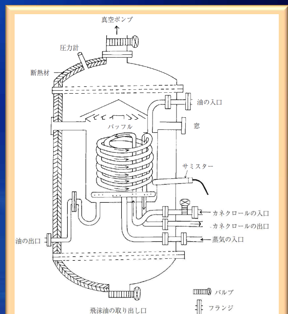
図 3.5. カネミ倉庫株式会社製油部ライスオイル精製工場の脱臭タンクの構造 (徳瀬化学工業株式会社提供の資料による)
