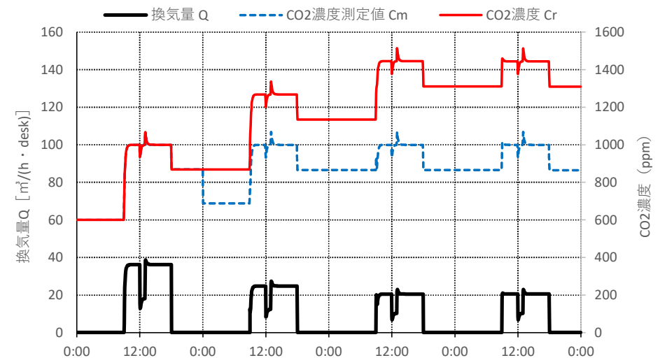
CO 2 濃度誤補正による換気不良の試算
