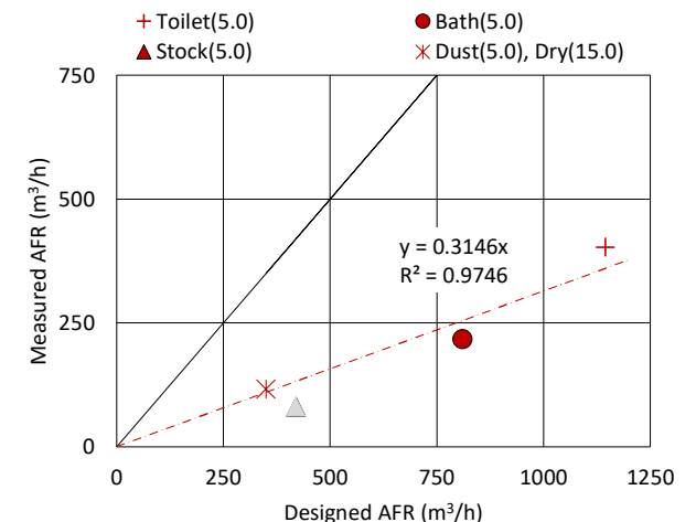
排気量の設計値と測定値
