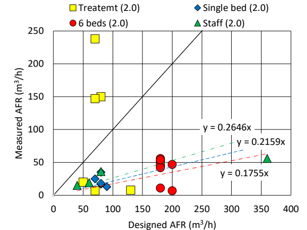
給気量(外気供給量)の設計値と測定値
