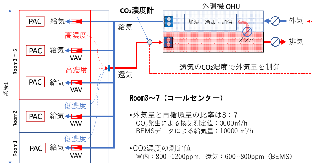
空調換気設備の概要と換気量の測定結果
