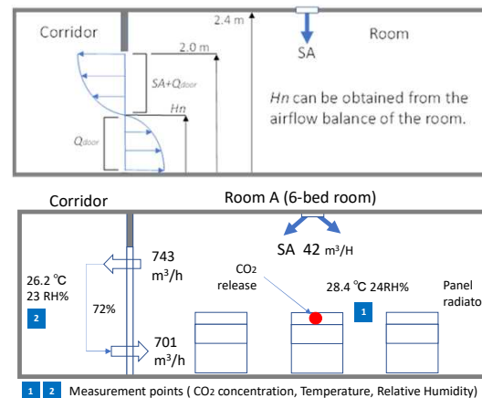
病室の換気と廊下への空気の流出
