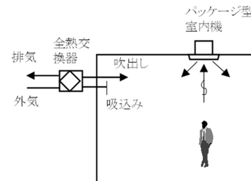
Bビルの空調・換気方式 (個別熱源・個別換気方式)
