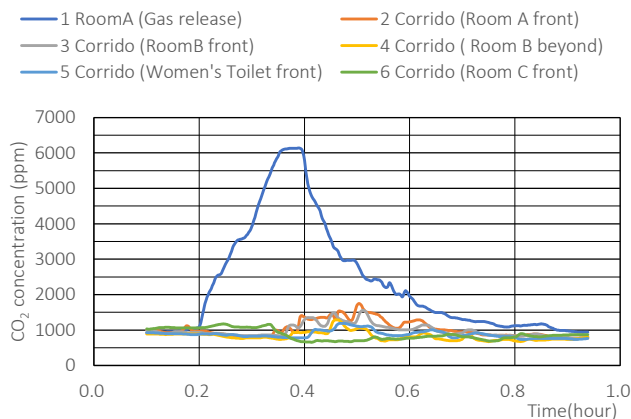
CO 2 濃度の応答
