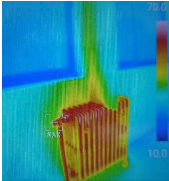
窓閉鎖時の温度分布
