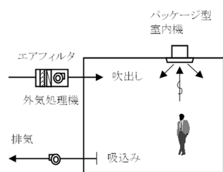
A, F, Gビルの空調・換気方式 (個別熱源・中央換気方式)
