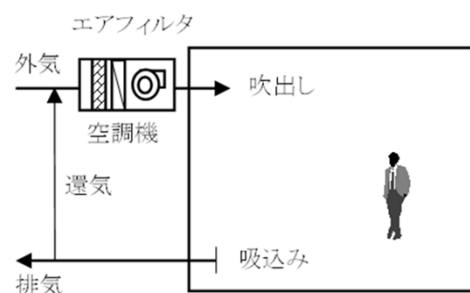
Cビルの空調・換気方式 (中央熱源・中央換気方式)
