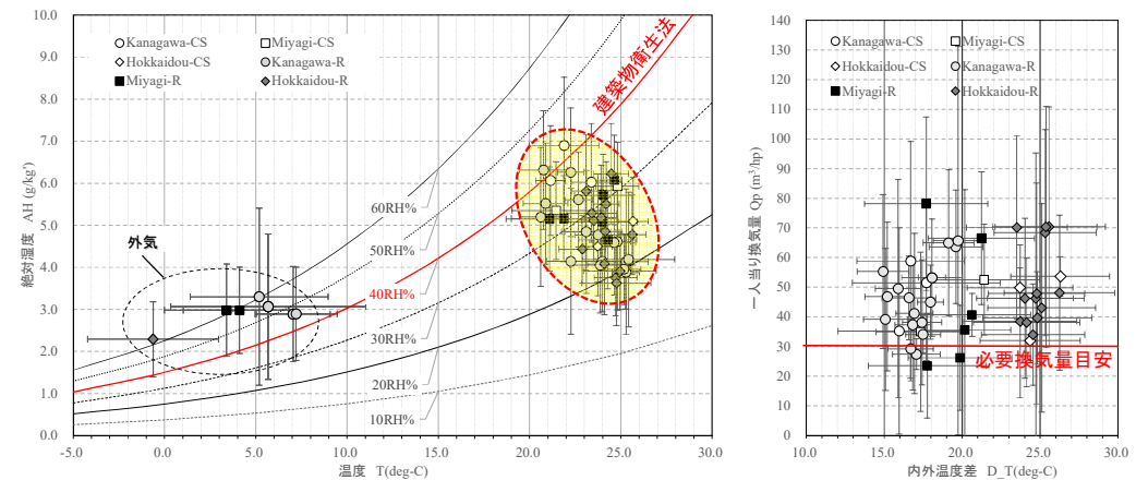
国内の高齢者施設の冬期室内空気環境(温度、湿度、一人当たり換気量)
