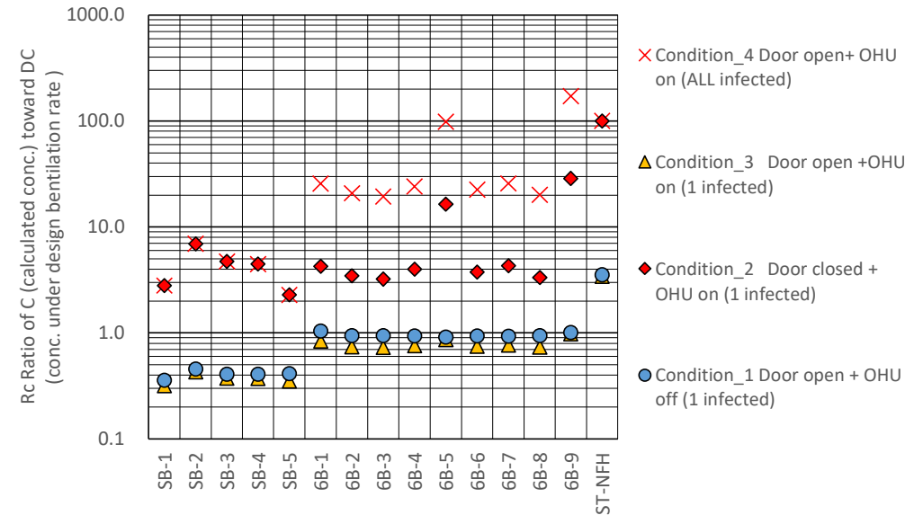
病室等の換気量減少による呼気濃度の上昇率
