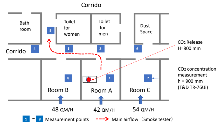
病室から廊下への空気の流出と廊下での移動
