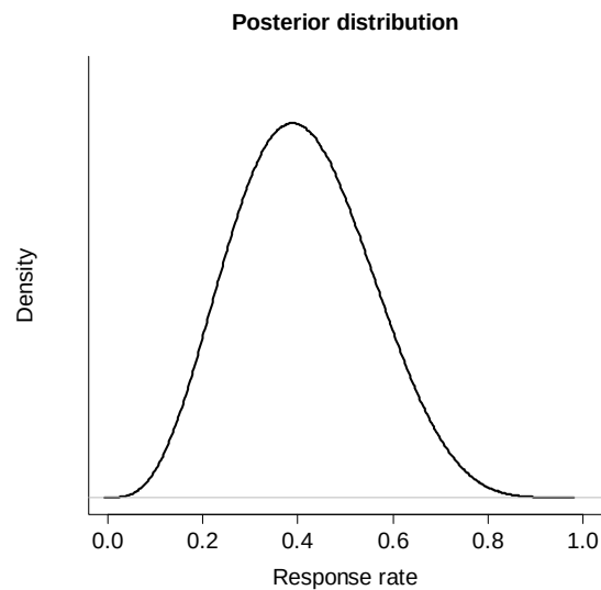
図1 奏効率 p_r の事後分布
