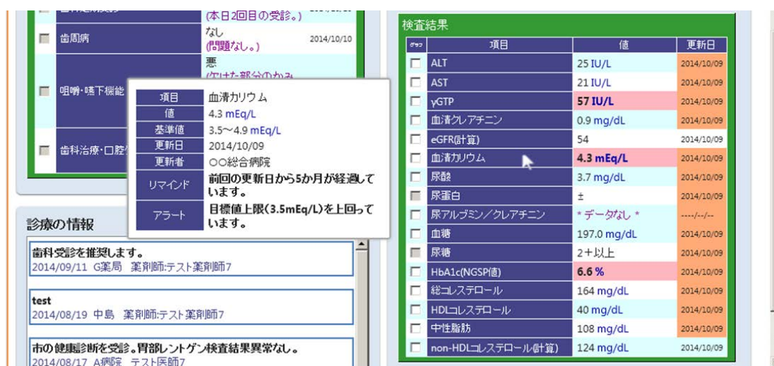
図 3.1-25 電子版疾病管理手帳アプリ（リマインド機能・アラート機能）
