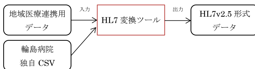
図 3.1-3 HL7 変換ツール
