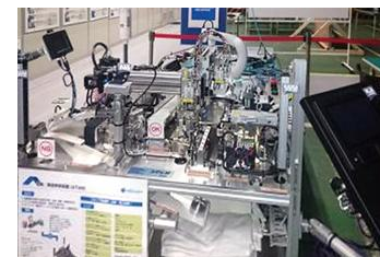
↑保全研修装置(AToM)
