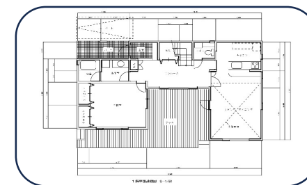
↑CADを使用して描いた建物の図面です。
