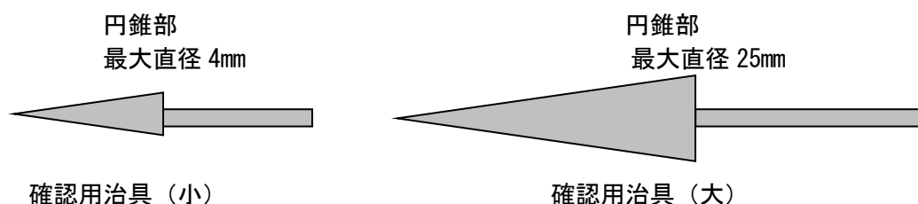
図1 可動部における指の挟み込みの確認用治具の例
