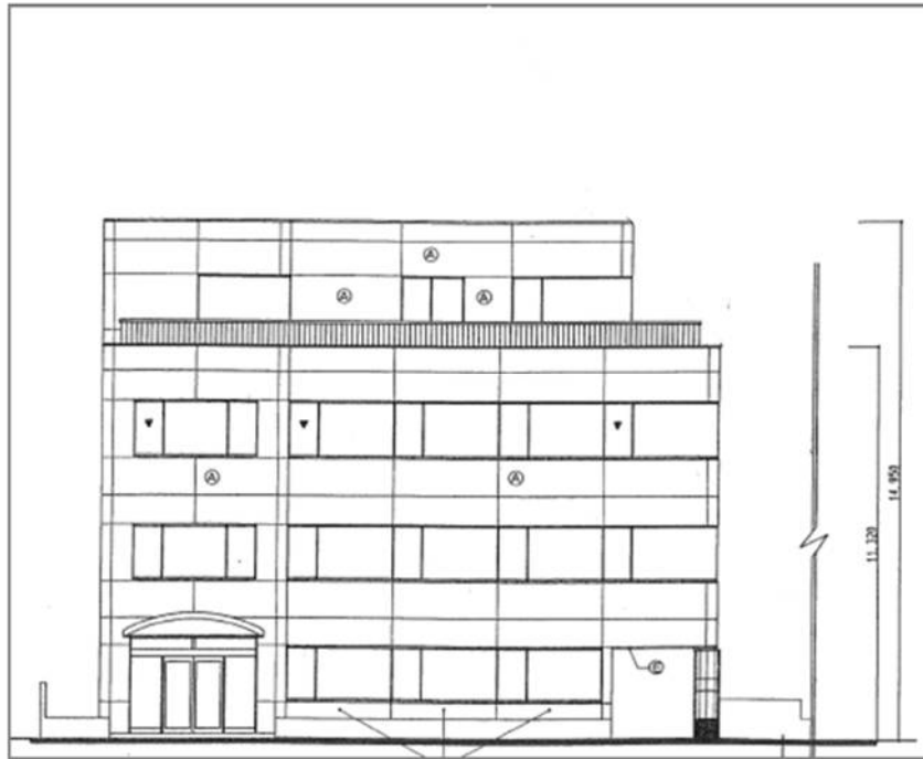
図 2.84 立面図
