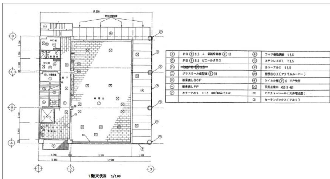
图 2.98 天井伏图
