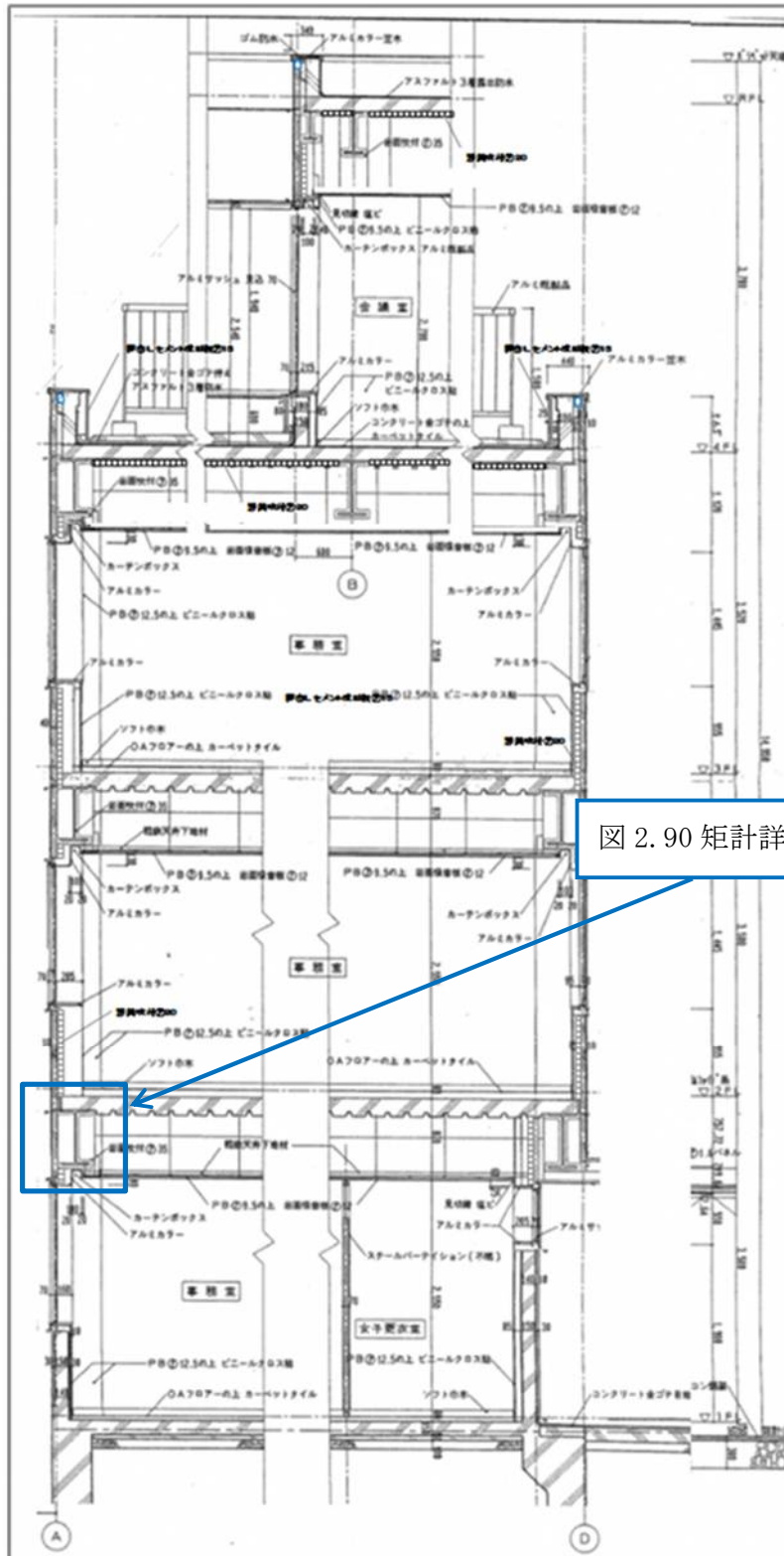
図 2.89 矩計図
