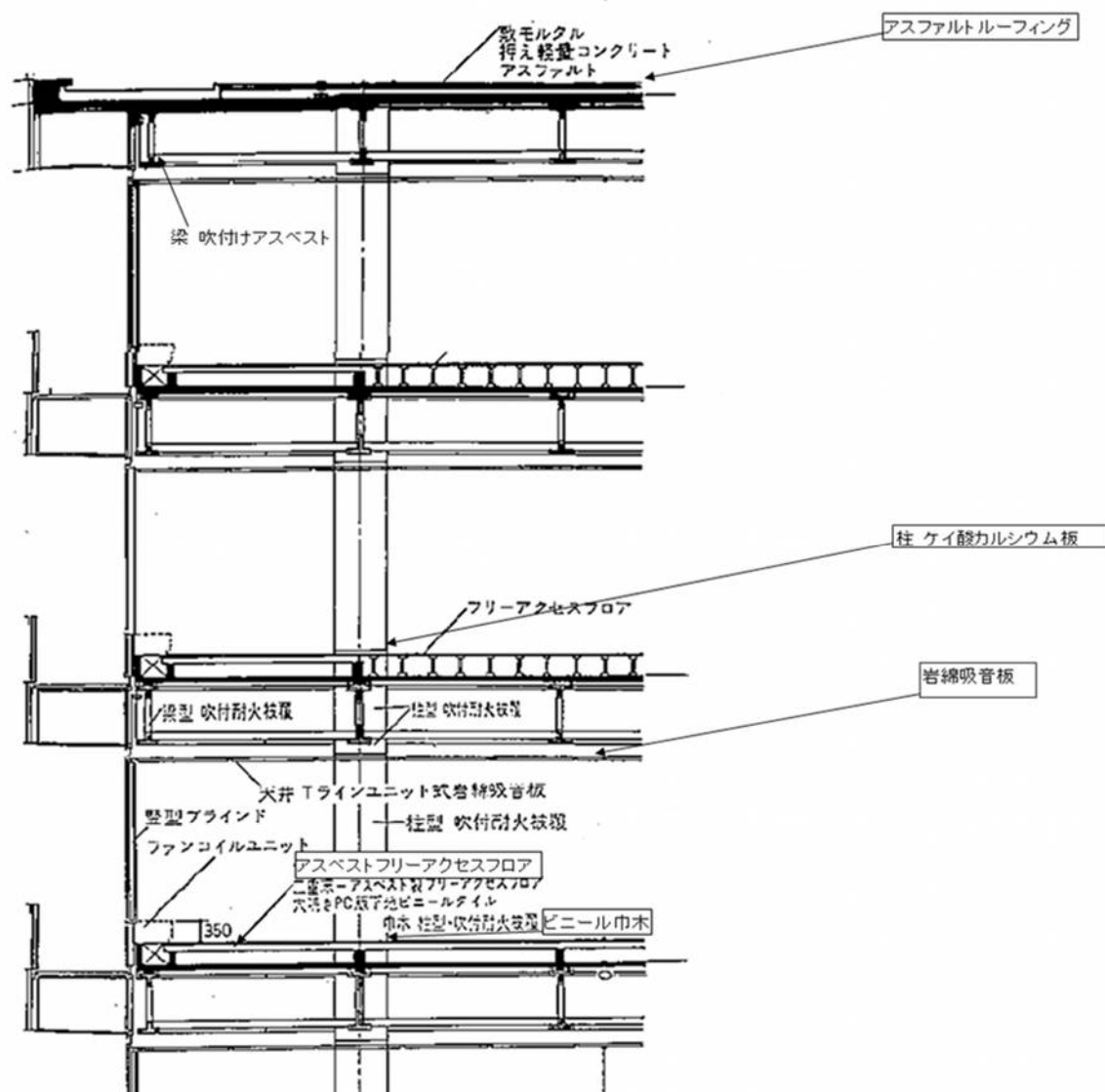
図 2.88 矩計図
