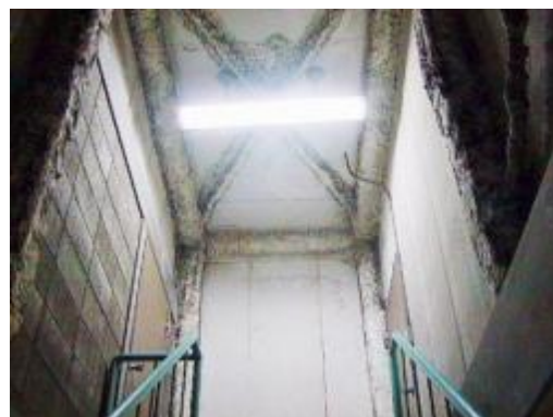
リプラス下地の吹付け RW、写真掲載ページに余裕があれば、組写真とした方がよい場合もある 階段室の防火区画で左壁のブロック上にラス網
