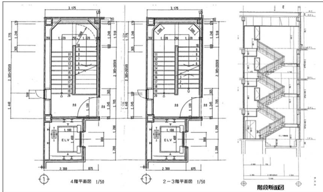
図 2.94 階段詳細図
