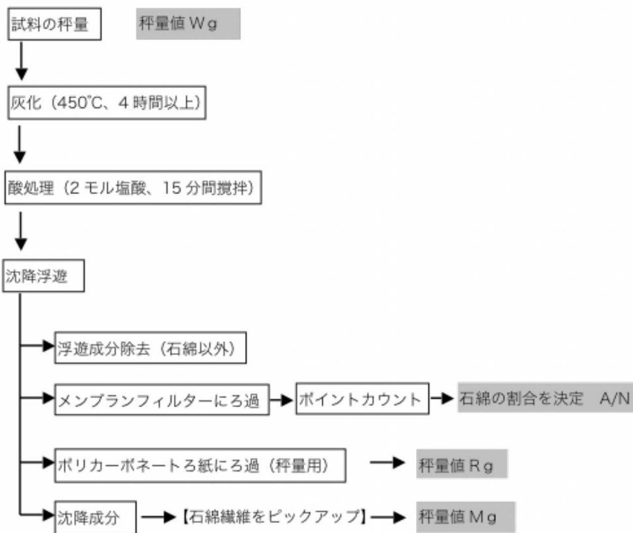
図 3.45 JIS A 1481-4 によるアスベスト含有率決定の手順の例
