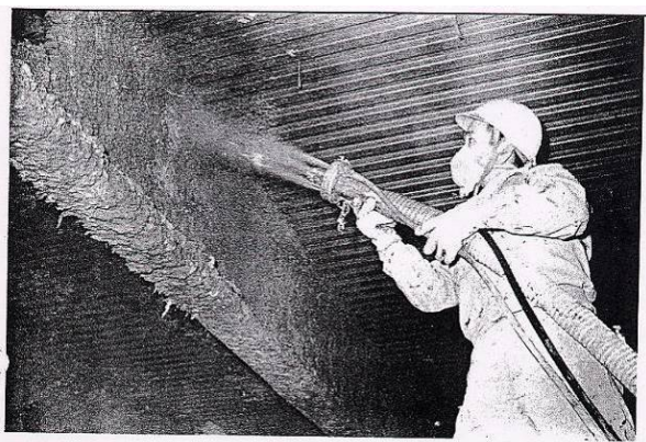
図 2.7 乾式吹付け施工と機械
