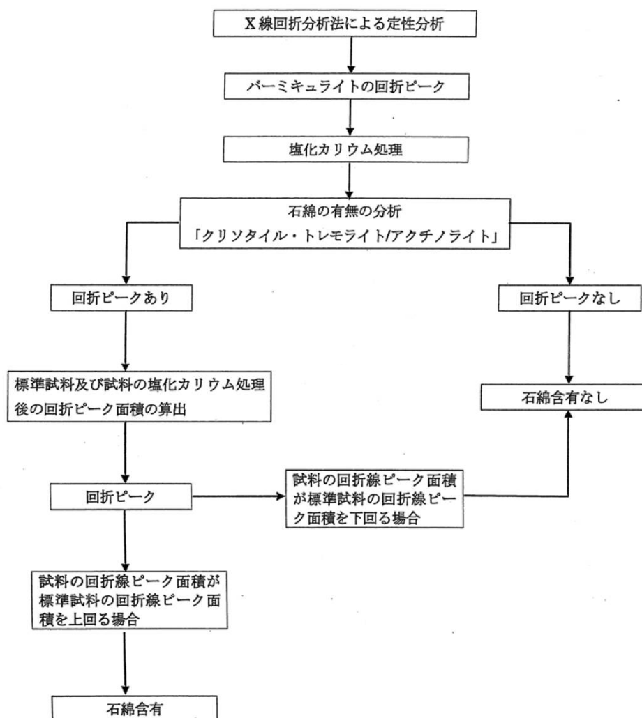
図 3.38 吹付けバーミキュライトの分析フロー
