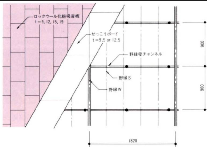
天伏図
