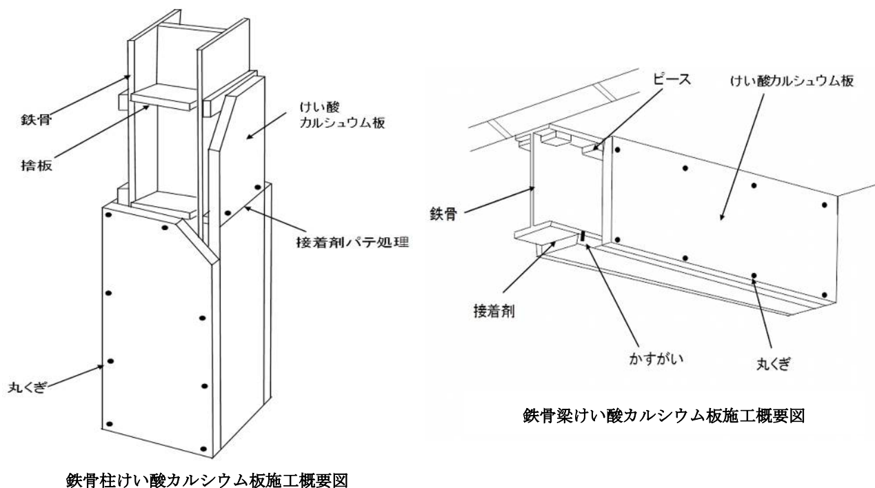
図 2.13 石綿含有けい酸カルシウム板第 2 種による被覆
