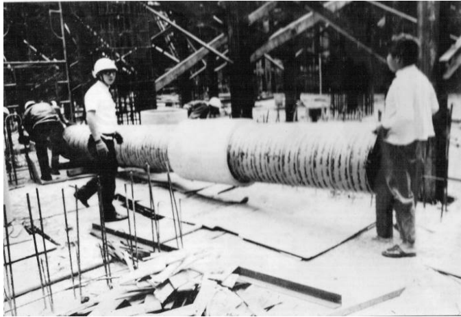
図 2.14 煙突用石綿断熱材の施工の様子
