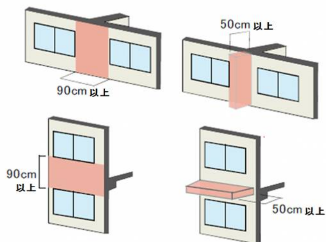
図 2.86 防火区画端部に接する外壁
