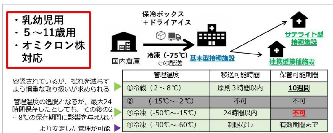
図 9 ファイザー社のワクチン（12 歳以上用以外）の配送・保管温度の関係
