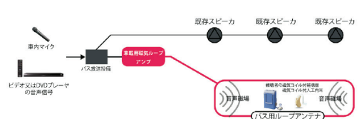
(右側) バス放送設備+磁気ループ設備
