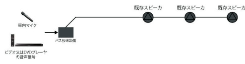
●バス放送設備システム系統図
