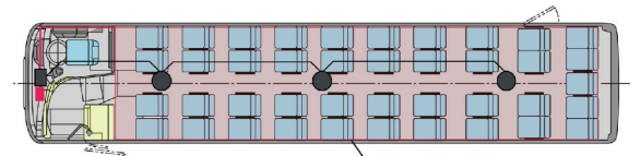
●バス放送設備+磁気ループ設備システム系統図
