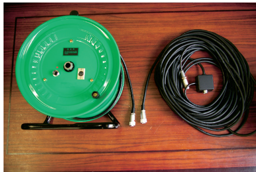
両磁気ループアンテナ (左側) 建造物用、(右側) 車載用
