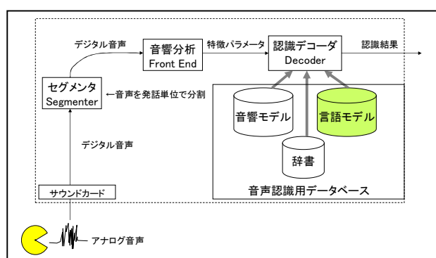
図3 音声認識のブロック図
