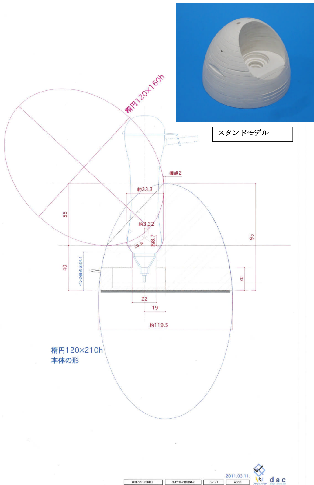
図 E-9 樹脂成形スタンド コンセプト&モデル
