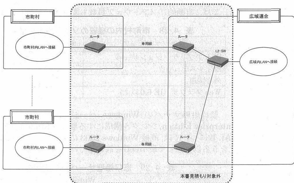
図 4・3 専用線構成図
