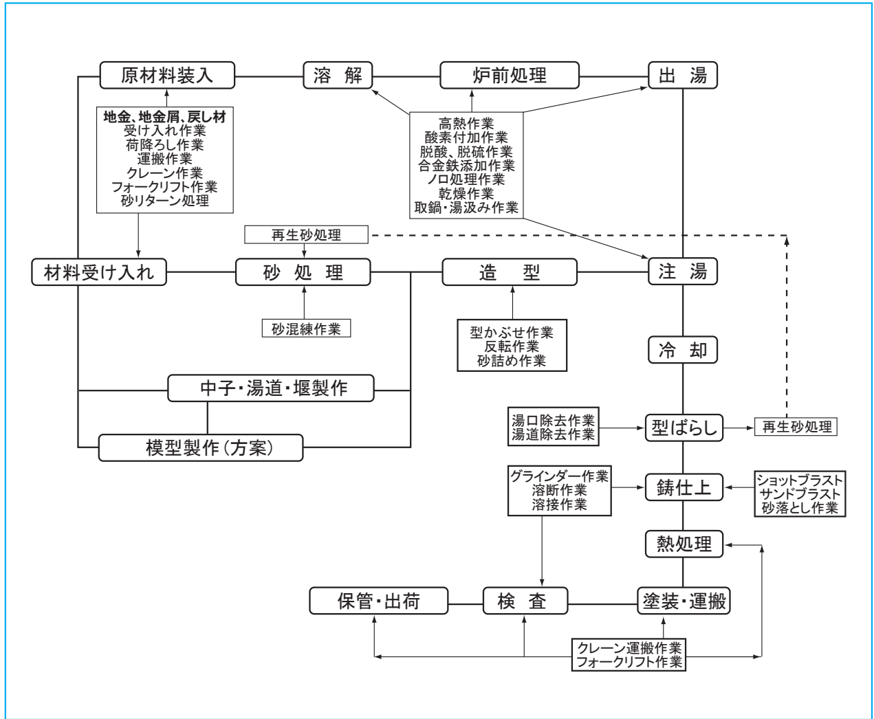
図 2 - 2 鋳物製造業の標準工程
