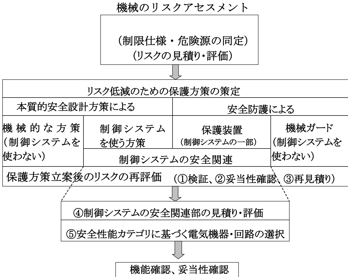
図26 一般的な機械部分と制御システムの安全関連部のリスクアセスメントの関係
