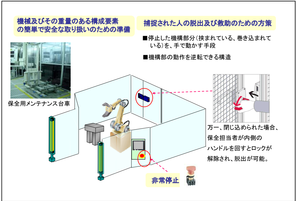
図 2 0 : 付加保護方策 (例)
