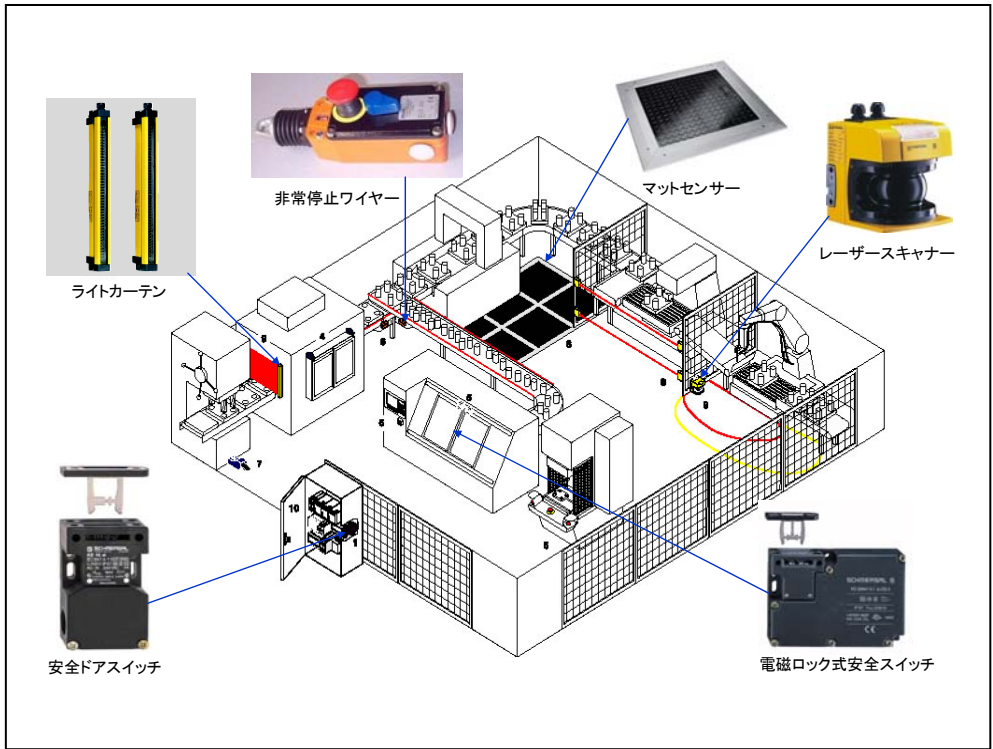
図 2 1 : 必要な安全防護及び追加の安全方策 (例)
