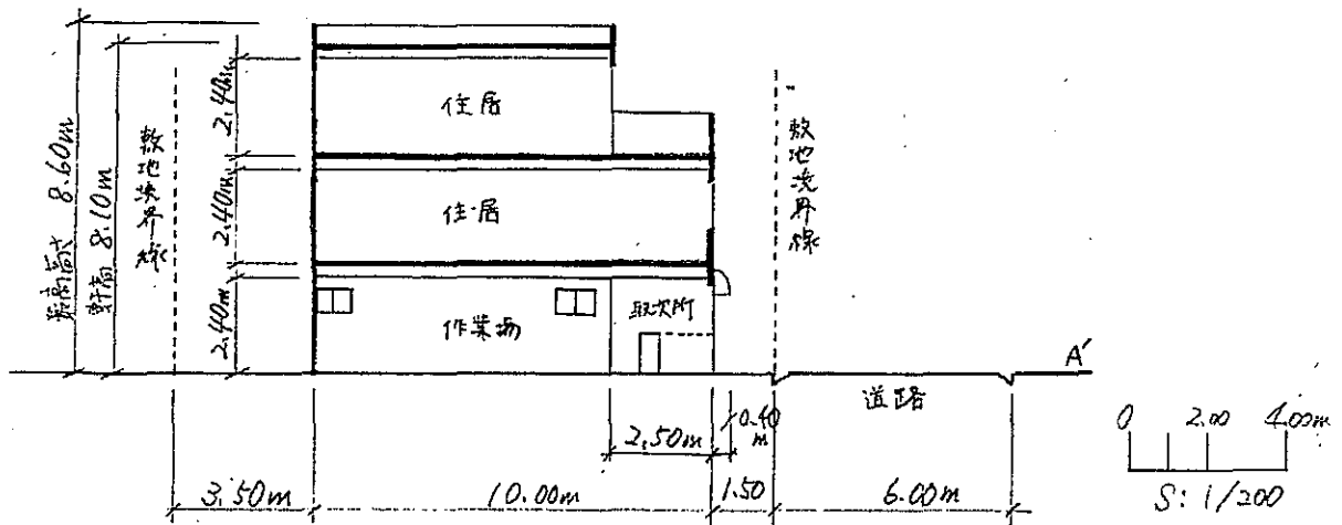
<B-B'断面图>
