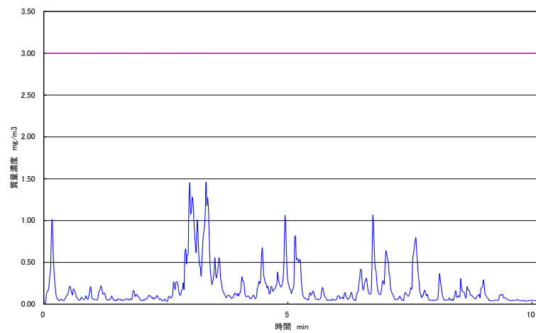
図 6.3 裁断作業(2回目)の裁断作業時のばく露濃度の時間的変動
