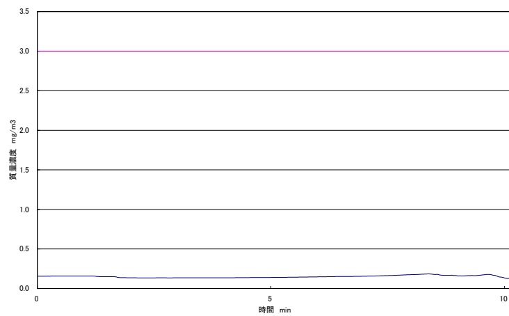
図 6.8 裁断作業(1回目)の裁断作業時のばく露濃度の10分間移動平均値
