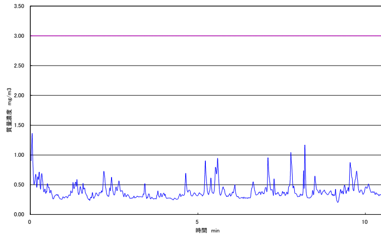
図 6.1 裁断作業(1回目)の裁断作業時のばく露濃度の時間的変動
