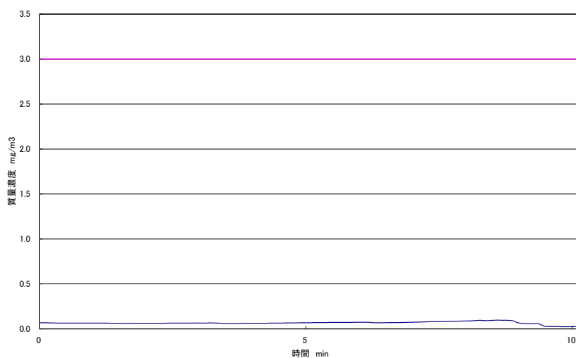
図 6.6 裁断作業(9回目)の裁断作業時のばく露濃度の10分間移動平均値
