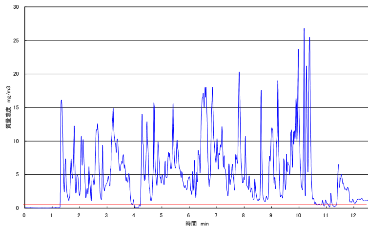
図 4.43 研磨作業(5回目)の研磨作業時のばく露濃度の時間的変動
