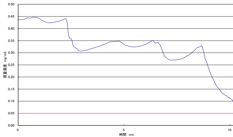
図 4.20 ばり取り作業(1回目)のばり取り作業時のばく露濃度の10分間移動平均値
