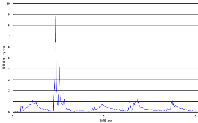
図 4.19 ばり取り作業(1回目)のばり取り作業時のばく露濃度の時間的変動
