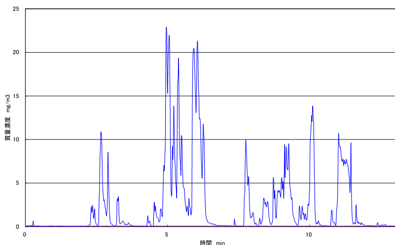
図 4.25 研磨作業(2 回目)の研磨作業時のばく露濃度の時間的変動
