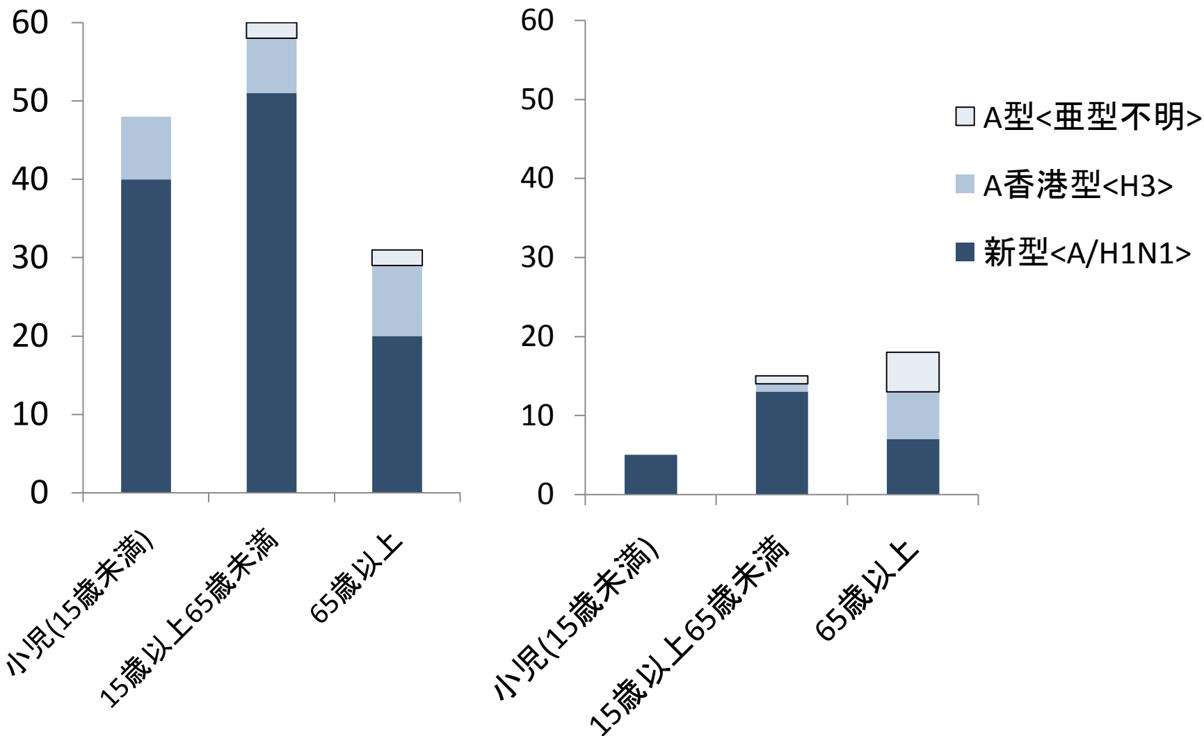
図9 重症患者における、PCR又は迅速検査で判明した亜型数(年齢階級別)
