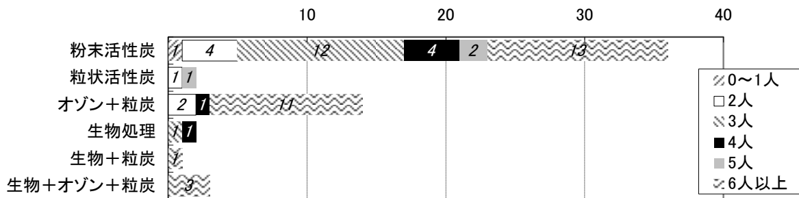
図-3-2-17 運転管理人数（平日昼間・施設能力 100,000 m³/日以上）
