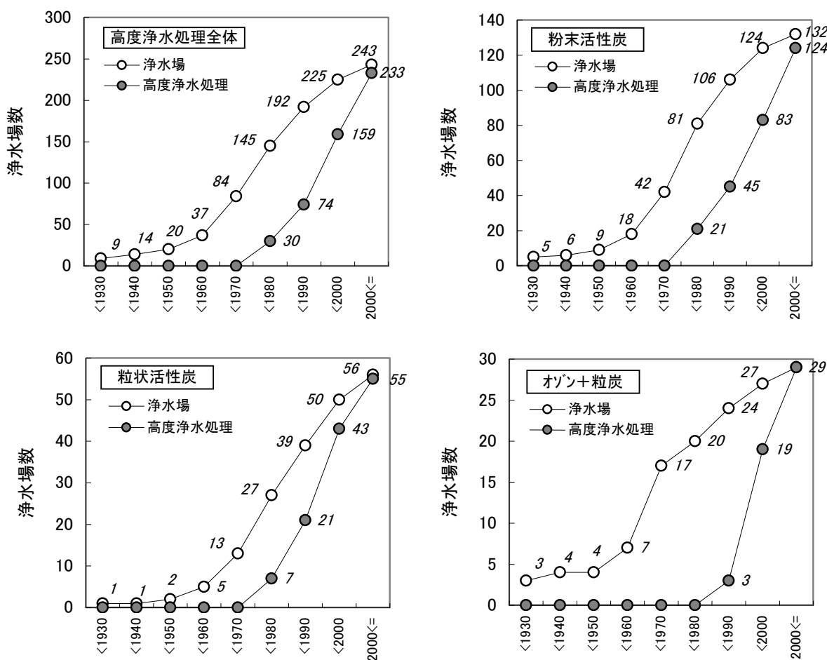
図-3-2-1 高度浄水処理を導入している浄水場における高度浄水処理施設の導入件数の経年変化 (1)
