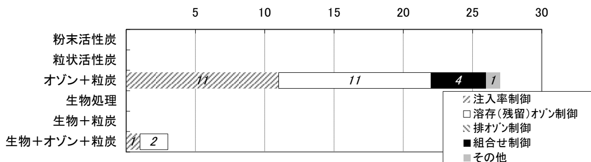
図-3-2-99 通常のおゾン制御方式
