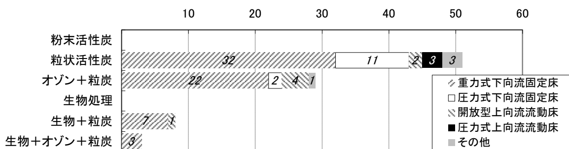
図-3-2-66 活性炭接触池の通水・炭層方式
