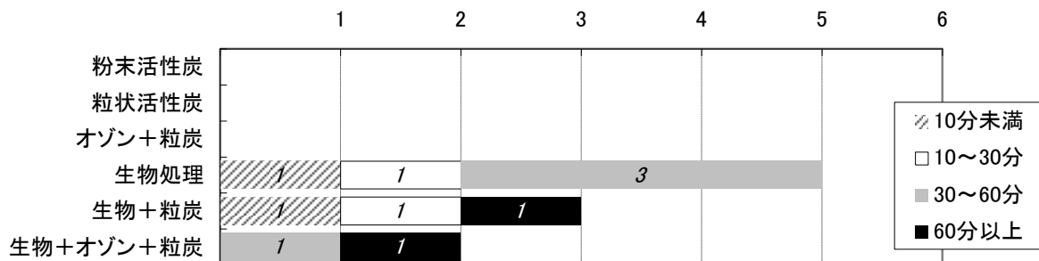
図-3-2-101 生物処理施設の接触時間
