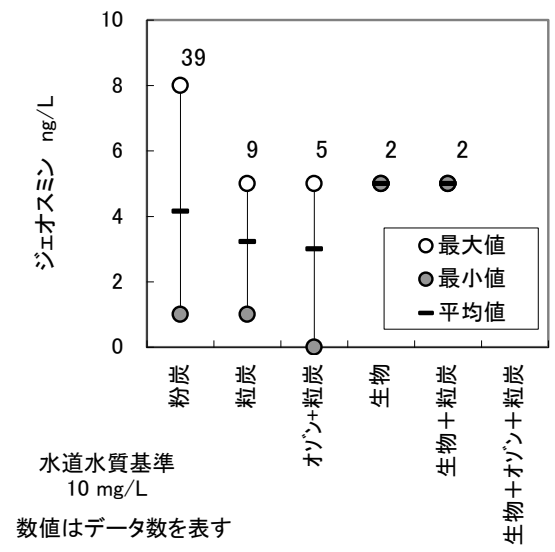
図-3-2-7 浄水水質の管理目標濃度 (2)
