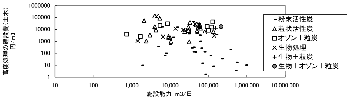
図-3-2-33 高度浄水処理の建設費（土木・単位水量当たり）
