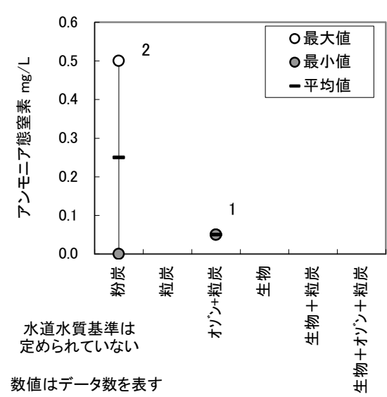
図-3-2-8 浄水水質の管理目標濃度 (3)
