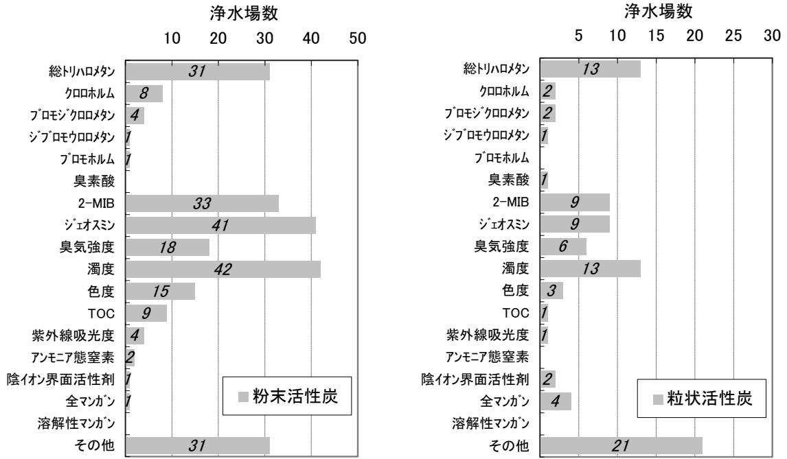
図-3-2-3 浄水水質の管理目標（水質項目（1））
