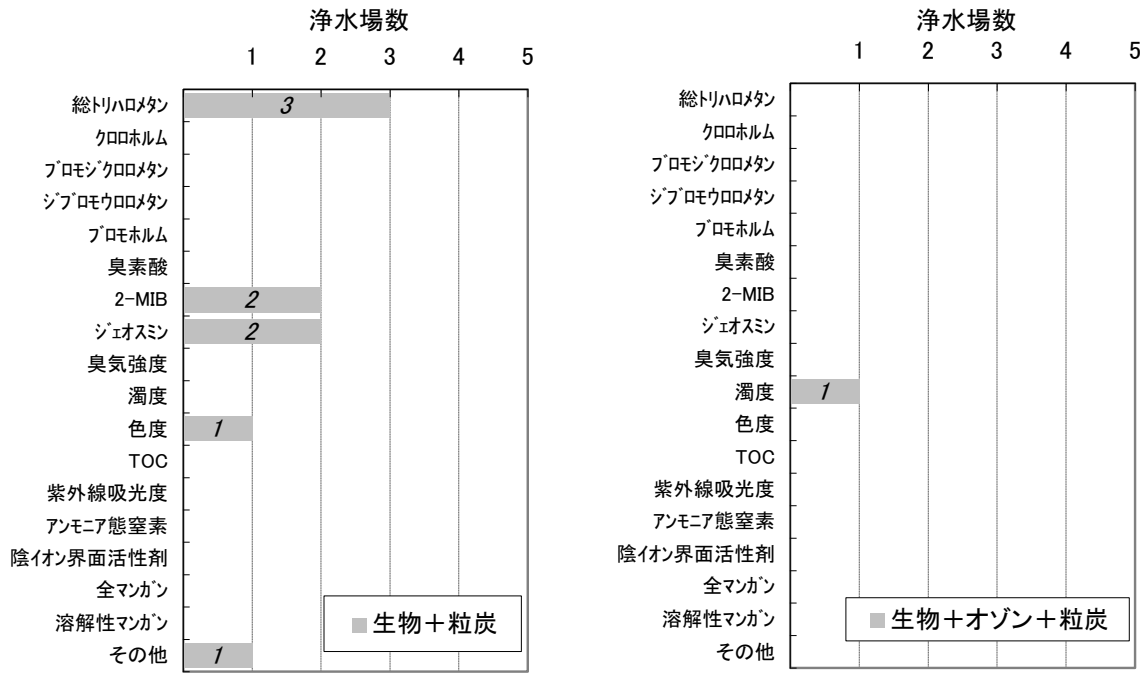
図-3-2-5 浄水水質の管理目標（水質項目（3））
