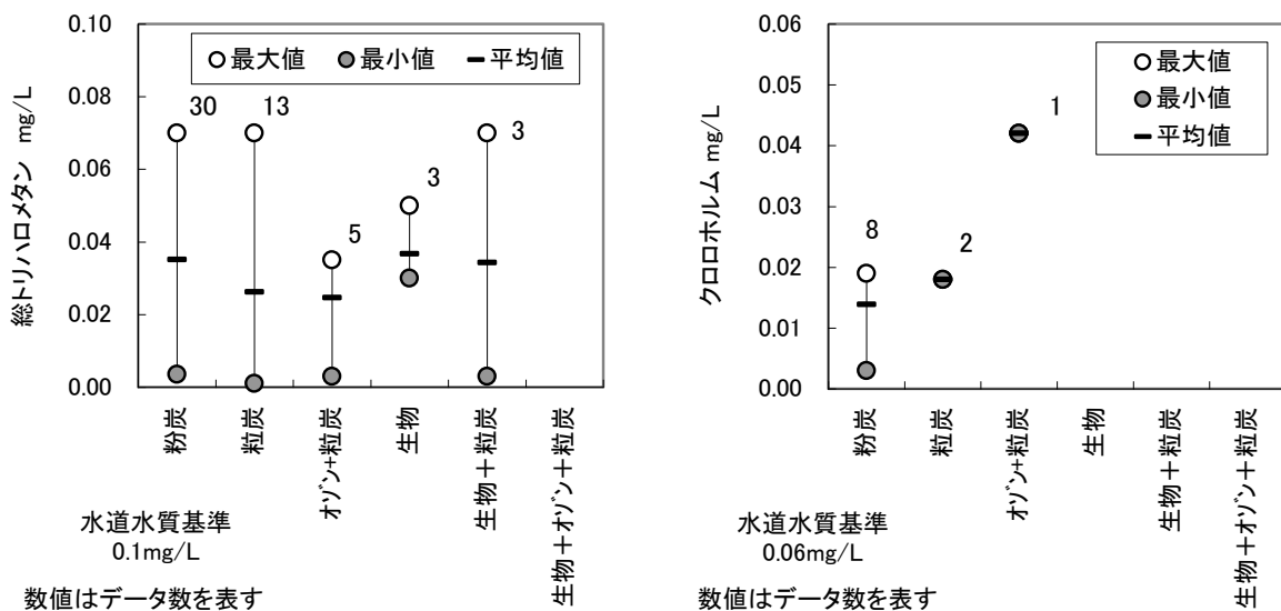
図-3-2-6 浄水水質の管理目標濃度（1）
