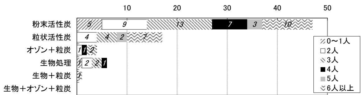
図-3-2-15 運転管理人数（平日昼間・施設能力 10,000~50,000 m³/日）
