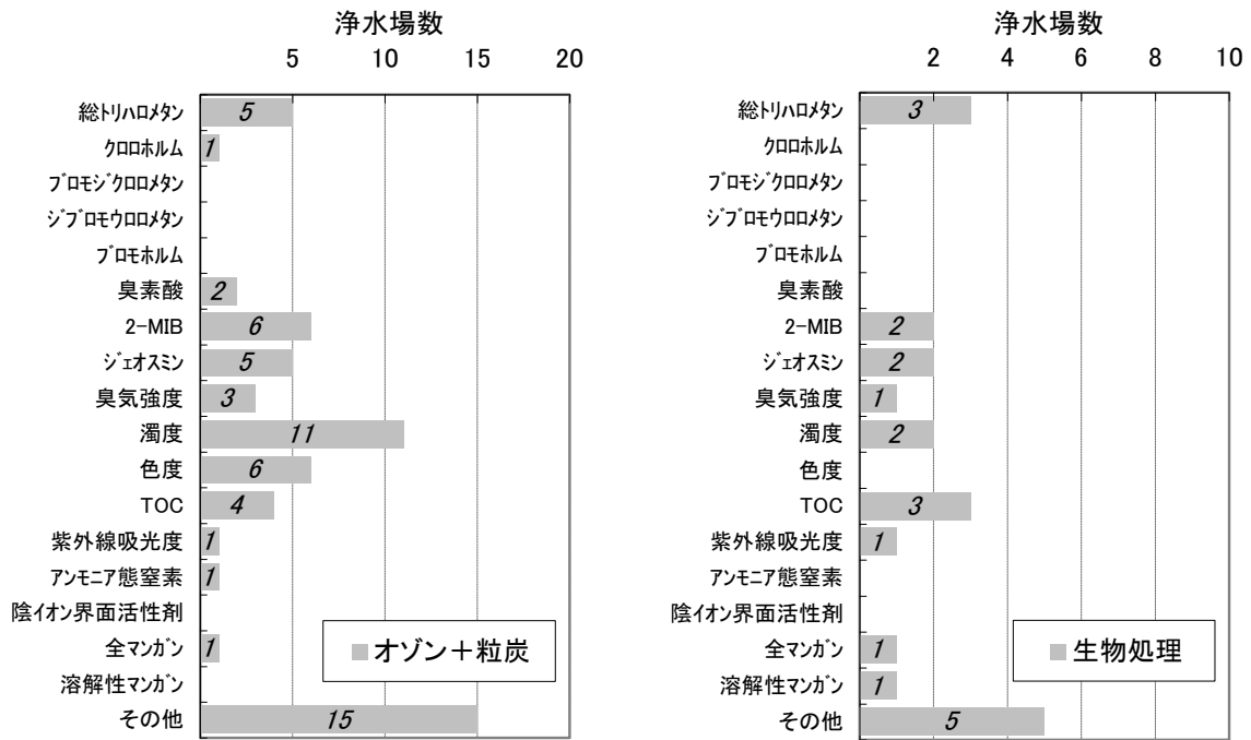
図-3-2-4 浄水水質の管理目標（水質項目（2））
