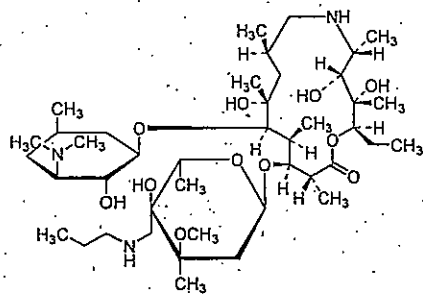
CP-472,295
